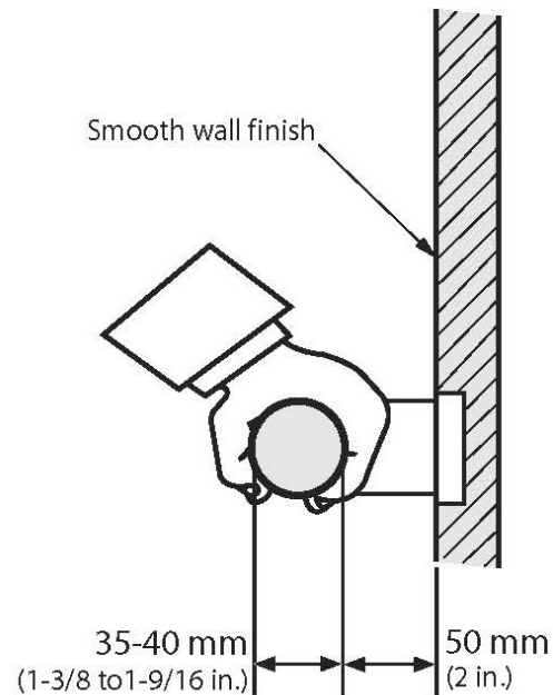
Figure 4.2.10.1 Grab Bar
