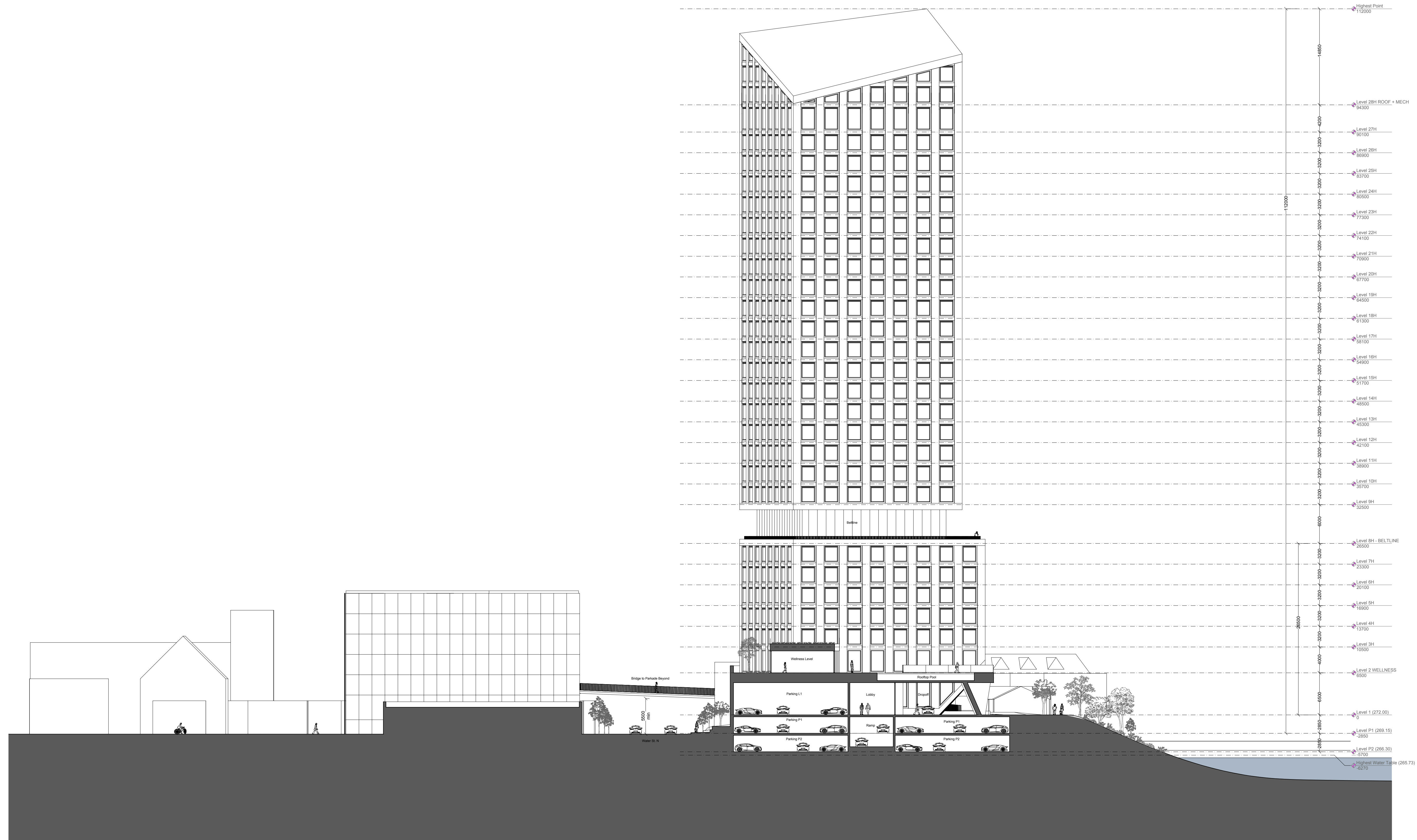
BB SITE CROSS SECTION B-B SCALE: 1:300
