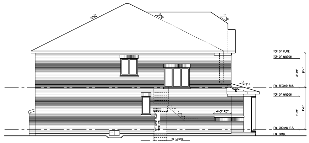
LEFT SIDE ELEVATION 'B'
